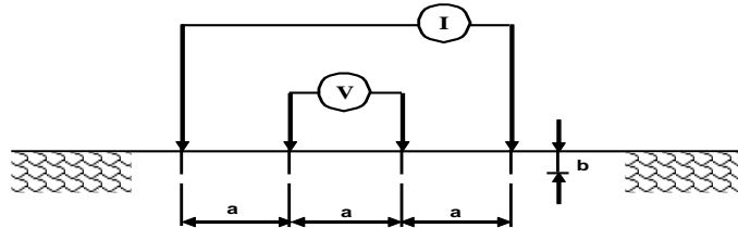
Figura 15.4. Esquema de medición de resistividad aparente
